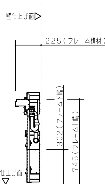
P 視図
