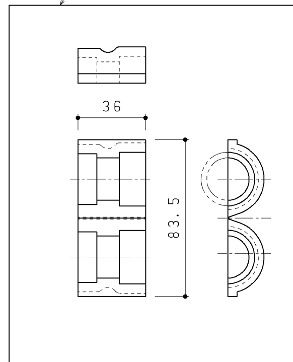
防露カバー(定流量弁部)
