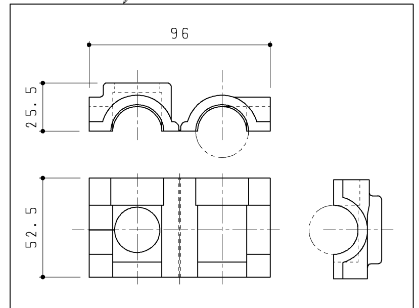
防露カバー(分岐金具部)
