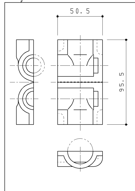
防露カバー(エルボ部、WL用)
