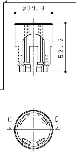
防露カバー(エルボ部、WL用)
