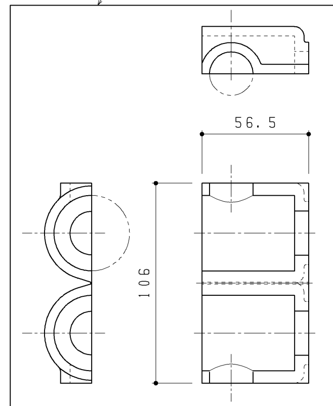
防露カバー(止水栓用)
