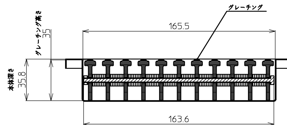
A-A' 断面拡大図(S=1/2)
