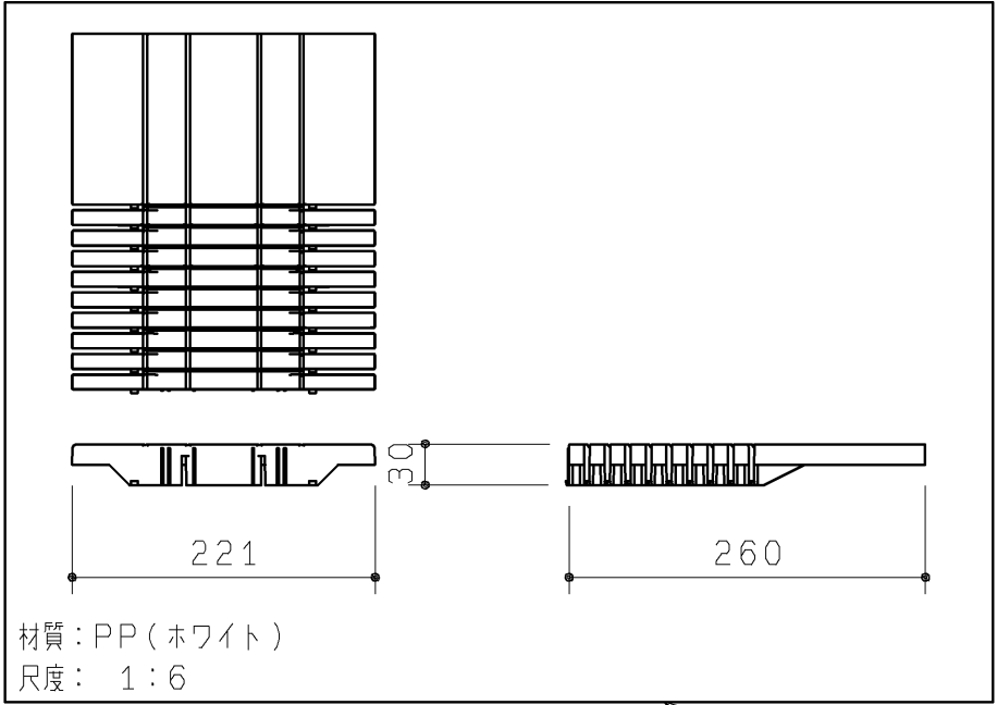
棚板(2ヶ)
