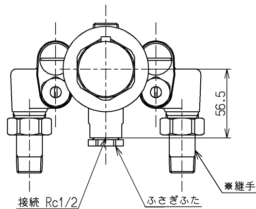
カバー取外し時の正面図
