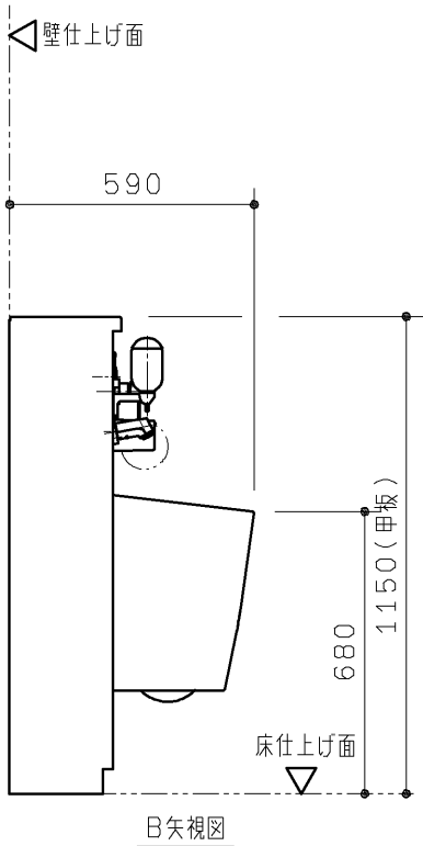
B矢視図
