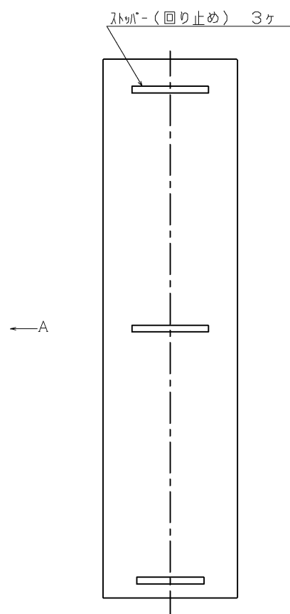
A 視 鏡止め金具、なべタッピンネジは除く。
