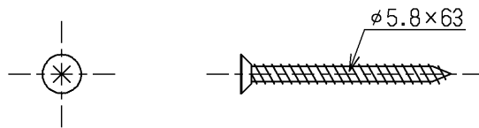
皿木ねじ(2ヶ):陶器取付け用
