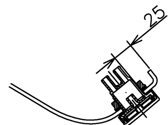
断面B-B(1:5)
