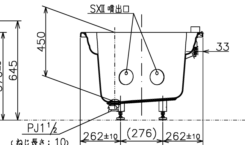
断面A-A
