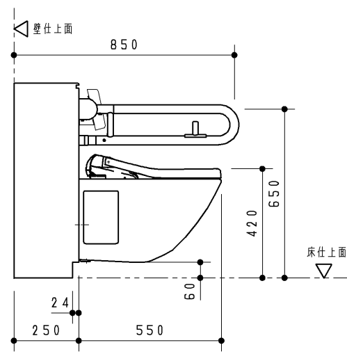
Q 視図
