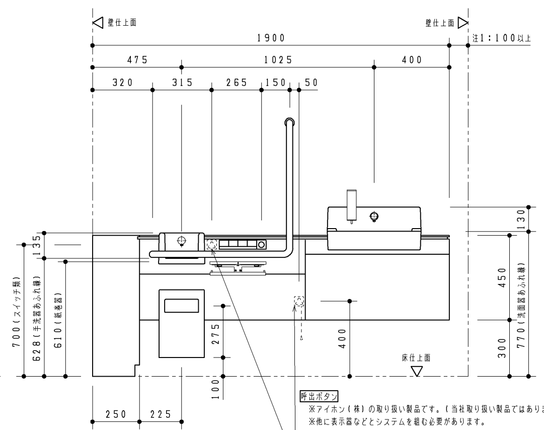
R 視図
