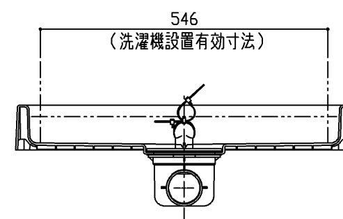
断面B-B
