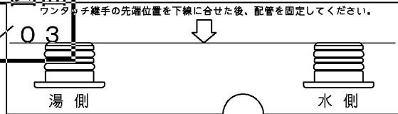
※部詳細図(1:2)
