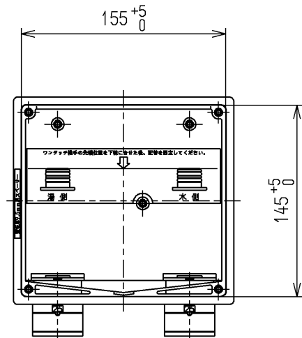
取付穴寸法(1:4)
