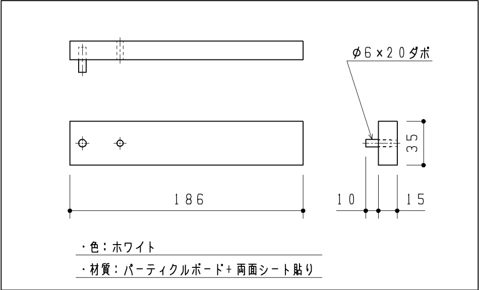
棚板受け材
