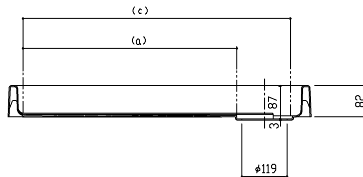
断面A-A
