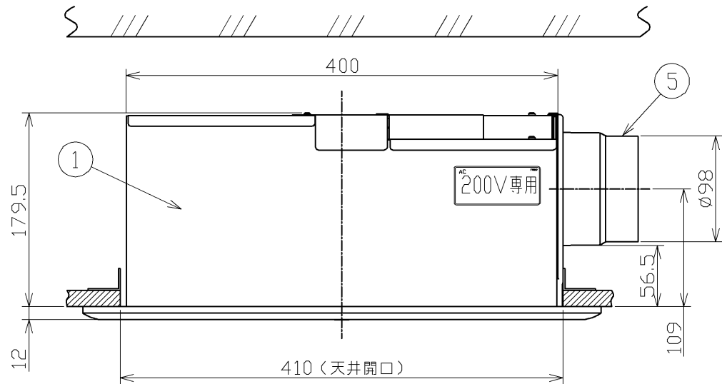
天井取付図 (1:5)
