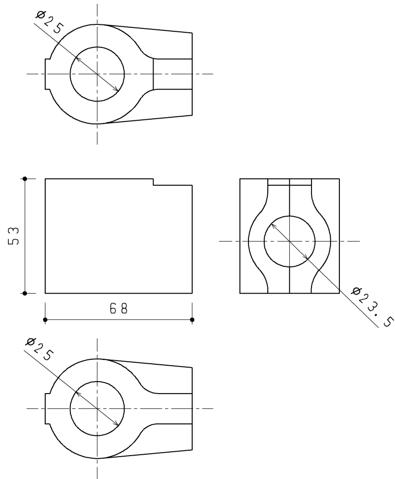
防露材（床給水短管用）
