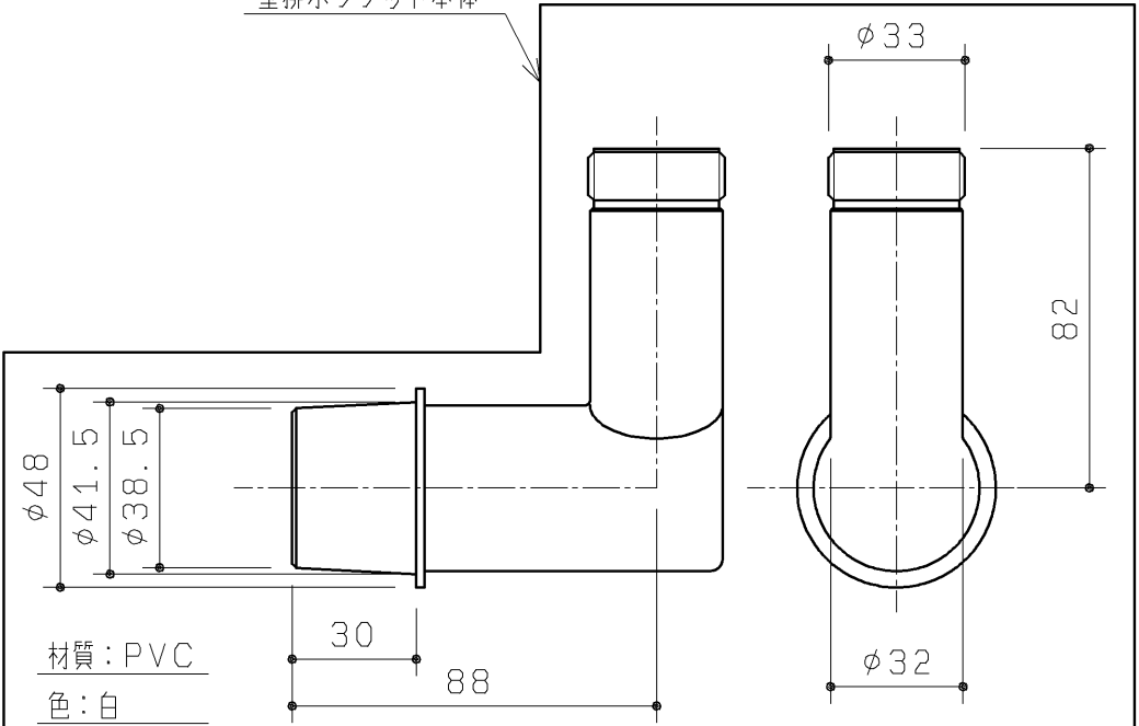
壁排水ソケット本体
