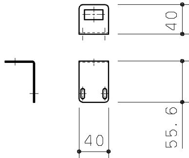
③ 側板中央固定材
