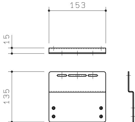
④ 側板下部固定材
