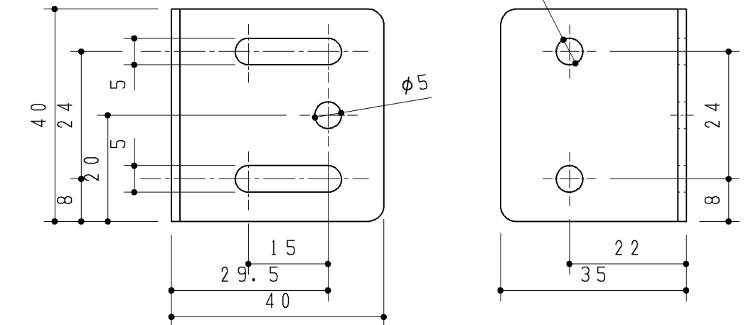
アングル材セット
