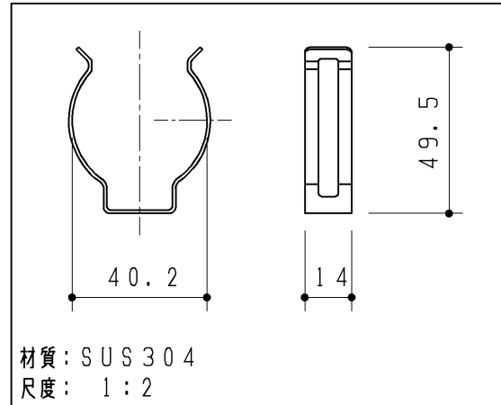
クイックファスナー
