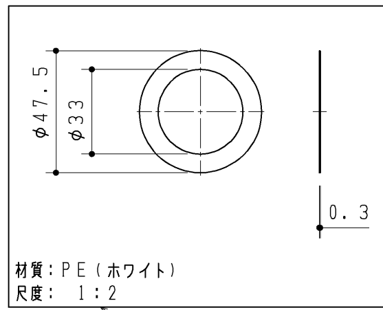
手洗器排水用スリップワッシャ
