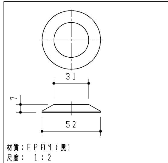
三角パッキン
