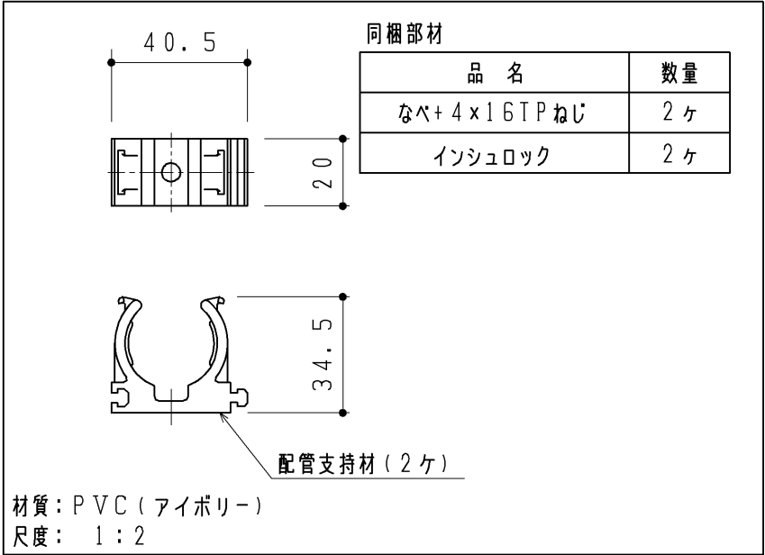
配管支持材セット
