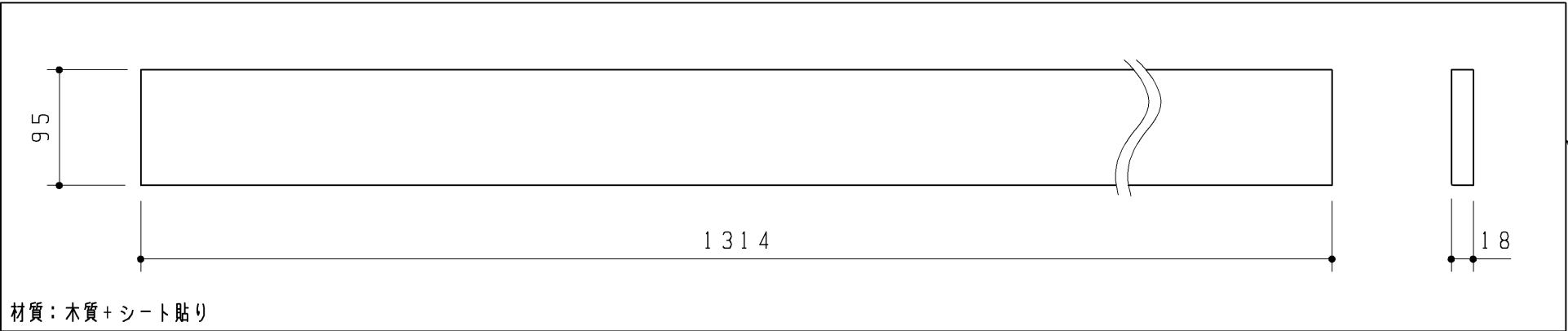
端部キャップ
