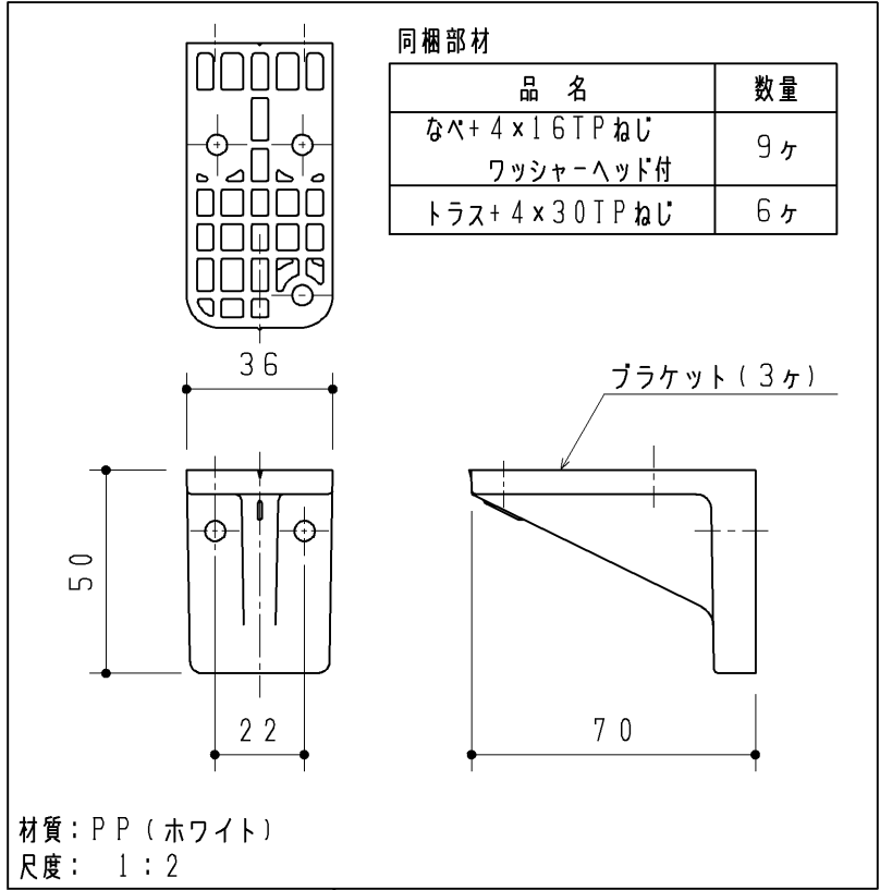
ブラケットセット
