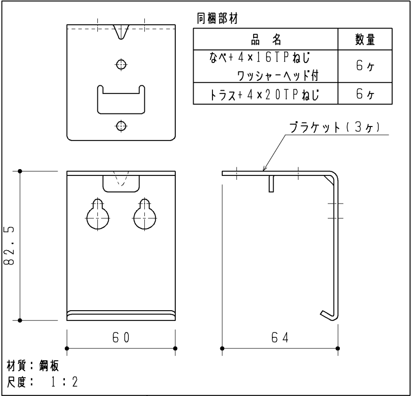
下段ブラケットセット
