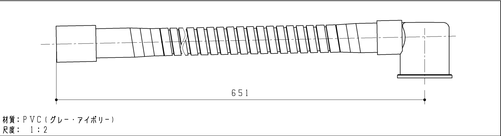
トラップ排水管セット
