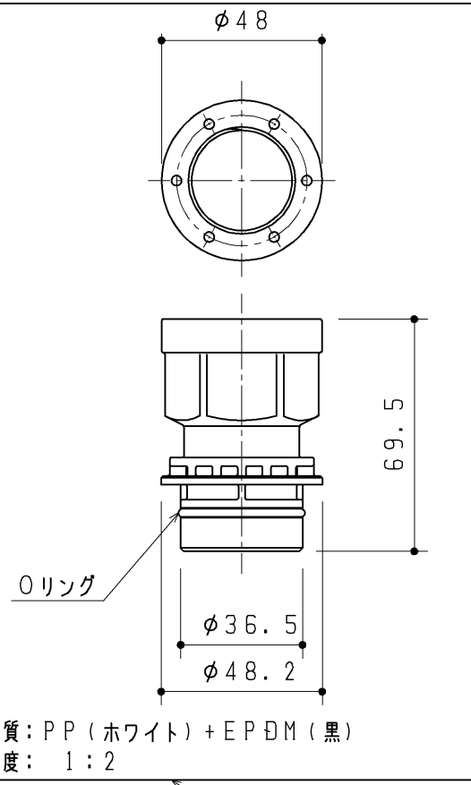
トラップ接続管
