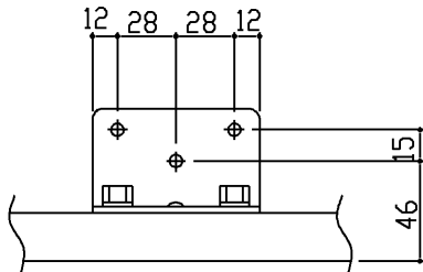
壁固定位置詳細（1／10）
