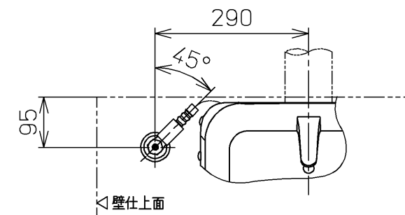
平面图
