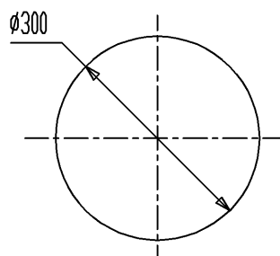
カウンター切込寸法
