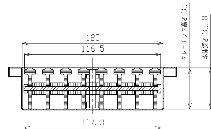
A-A断面詳細図 (1:2)
