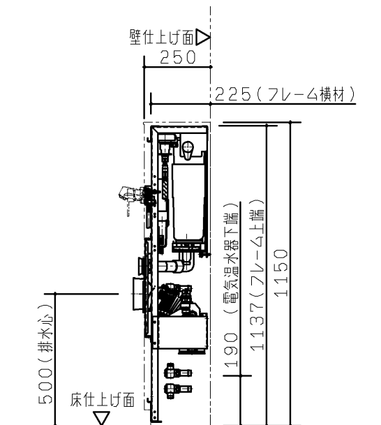
R 視図
