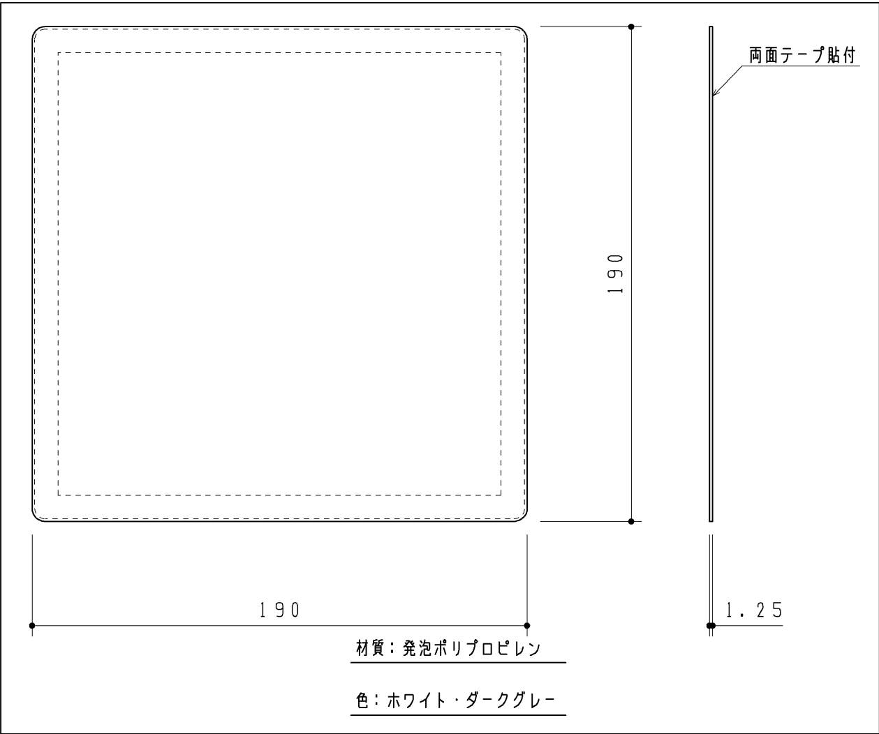
カバー（1ヶ）
