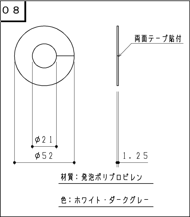
カバー（1ヶ）
