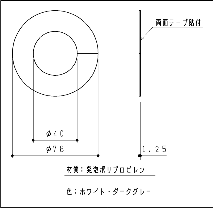
カバー（1ヶ）
