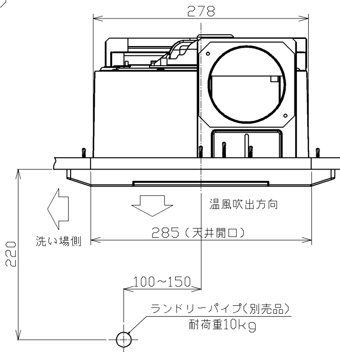
天井取付図 (1:5)
