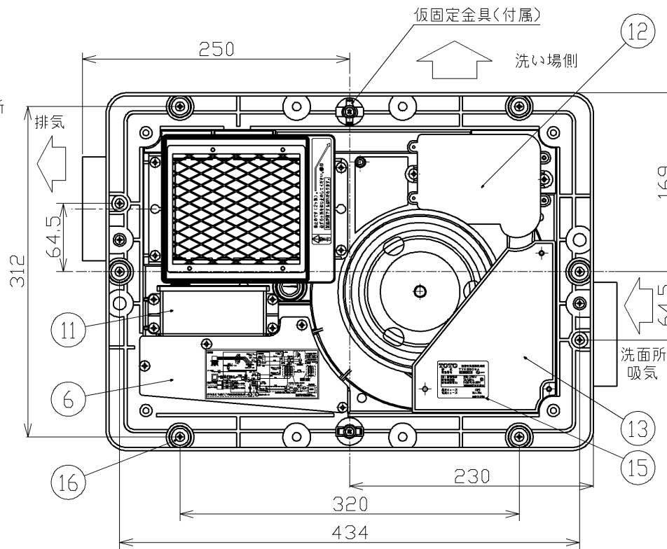
天井取付図 (1:5)
