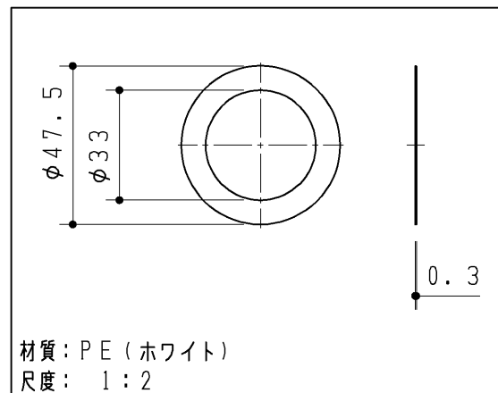
手洗器排水用スリップワッシャ
