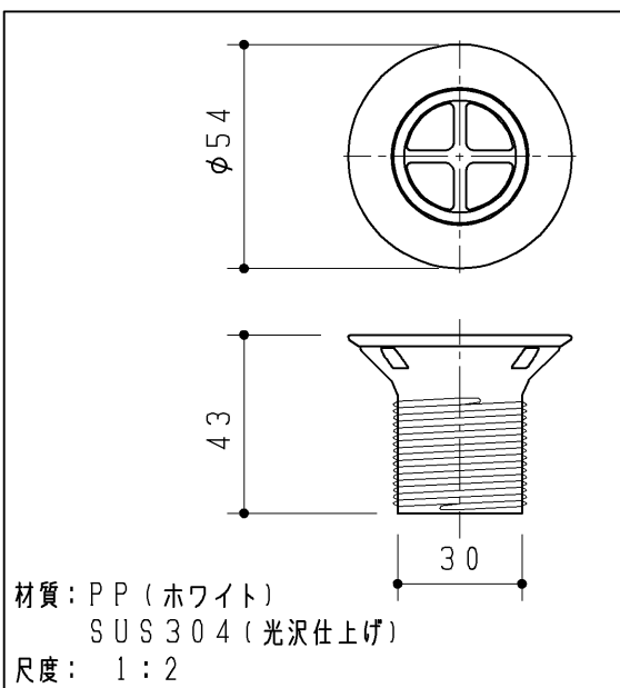
排水金具
