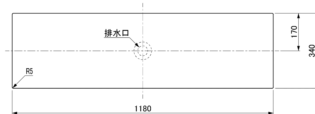
カウンター切込寸法
