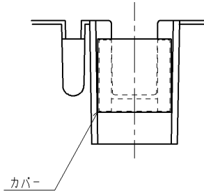
B 視図
