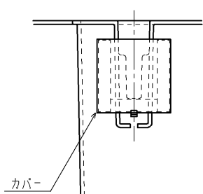
A 視図
