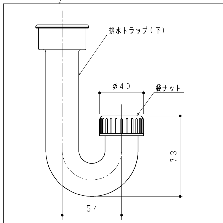
排水トラップ (下)
