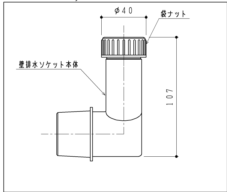
排水トラップ (下)
