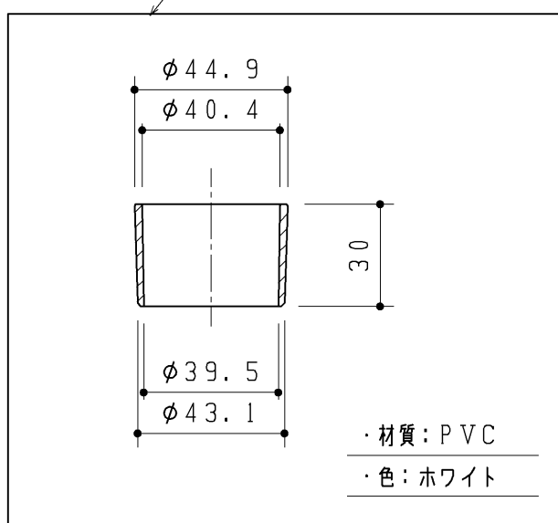
排水アダプター
