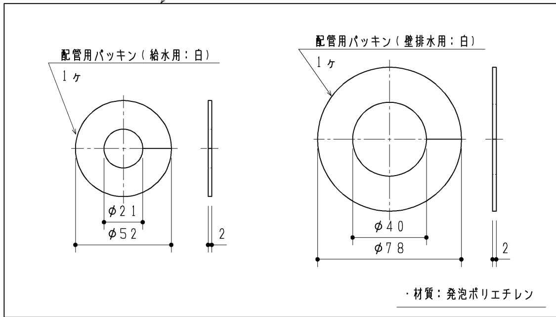
配管用パッキンセット (壁排水用)
