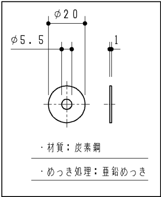
平座金 2ケ
