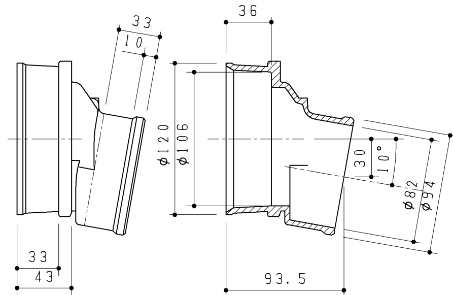
A-A断面図
