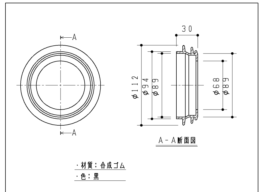
排水パッキン
