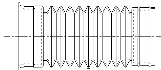
排水ソケット
