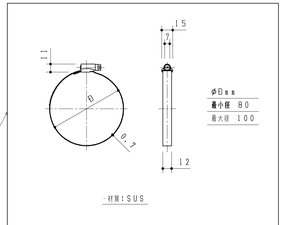
ホースバンド (2ヶ)
