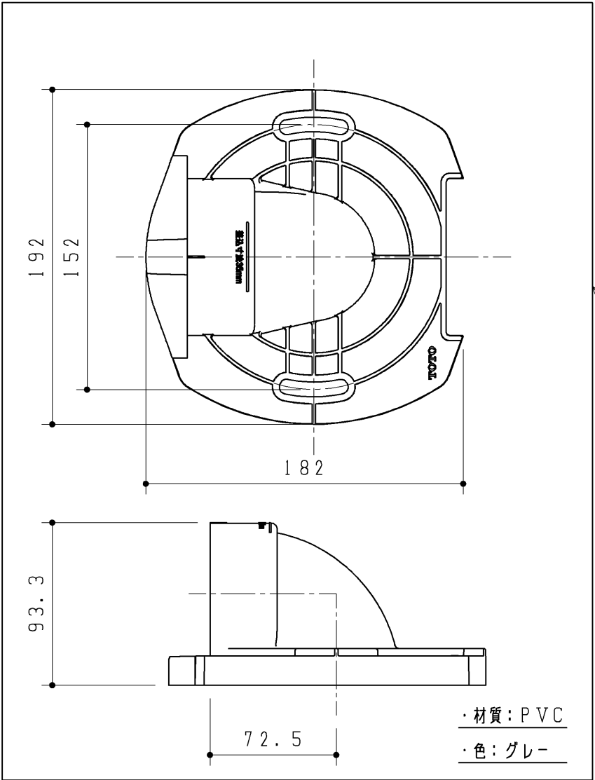
フランジ接続部
