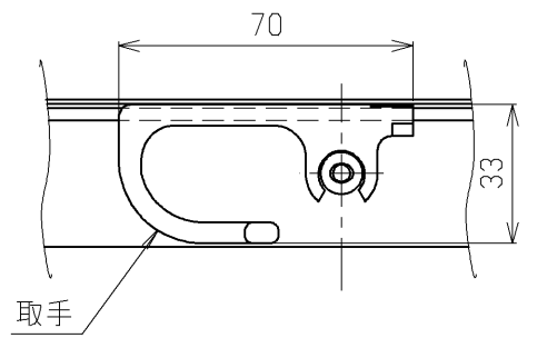
B-B断面詳細図 (1:2)
