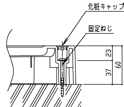
固定部詳細(尺度フリー)
