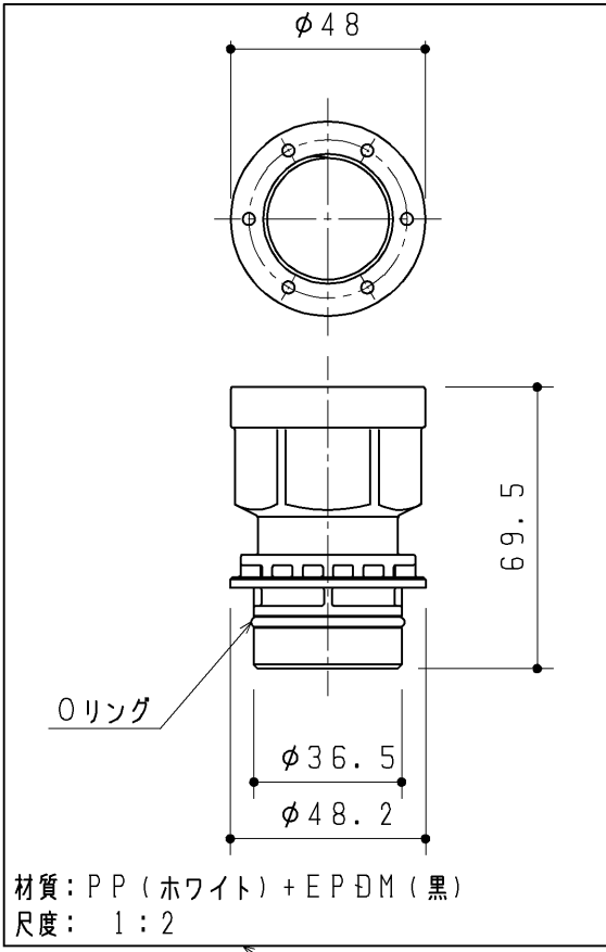
トラップ接続管
