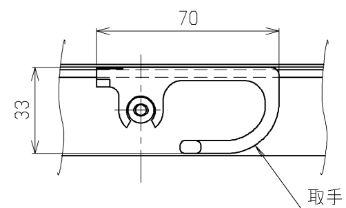
B-B断面詳細図 (1:2)
