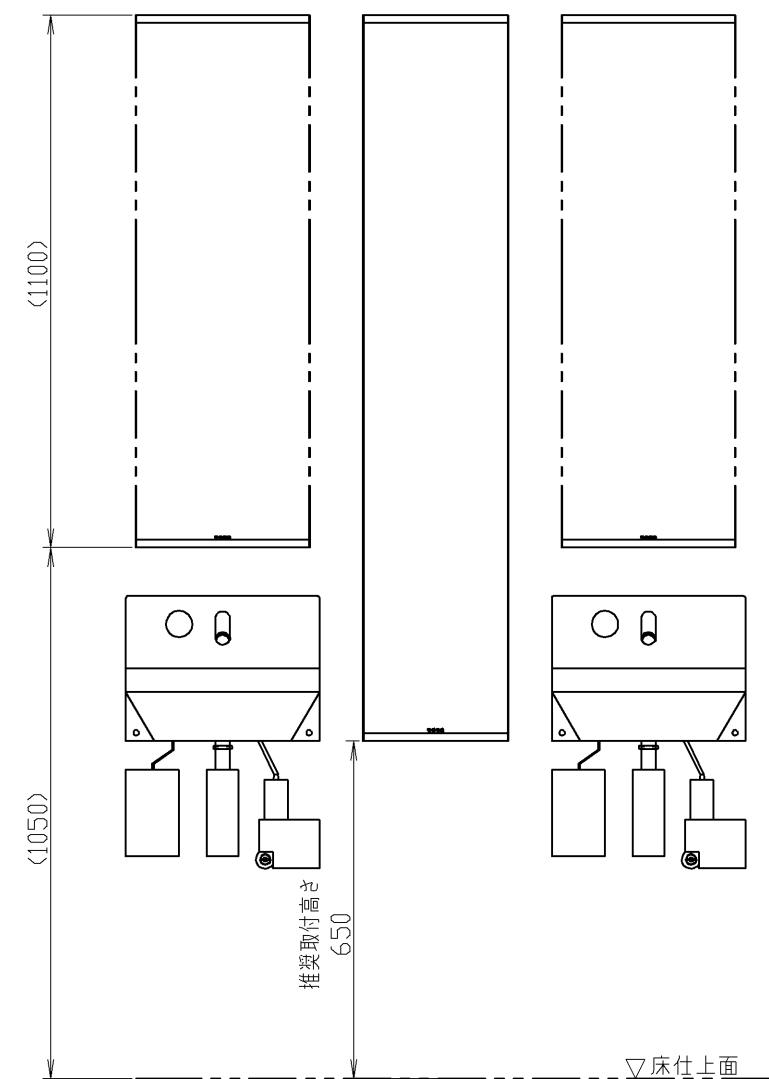
ニューラバトリースペース（棚なし）の場合の推奨取付位置
