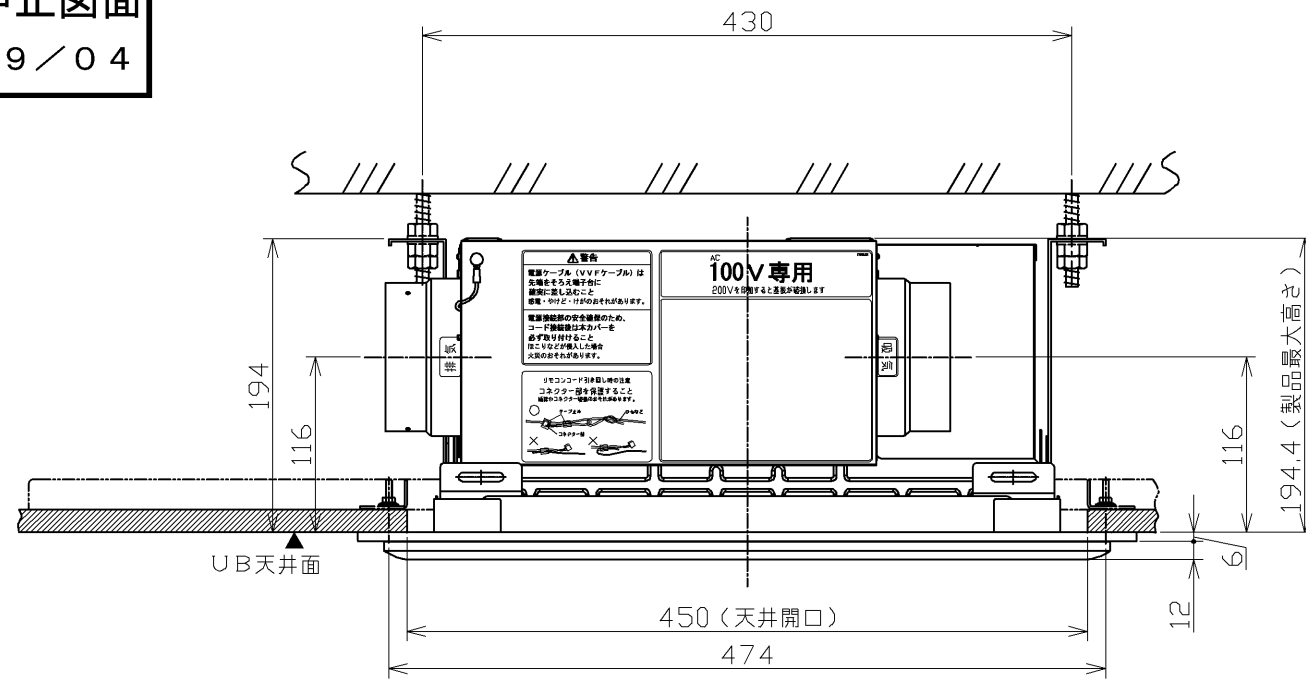
天井取付図
