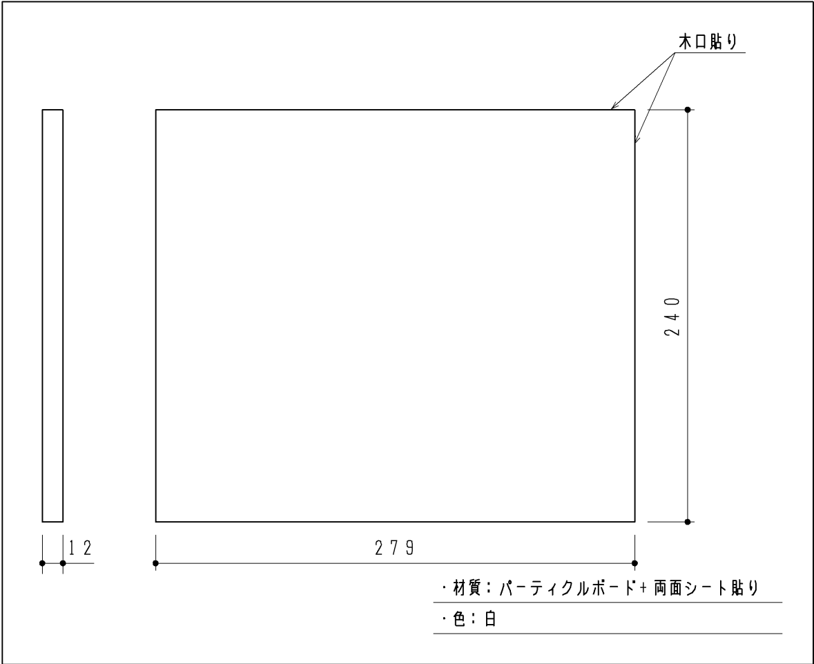
棚板 1ヶ
