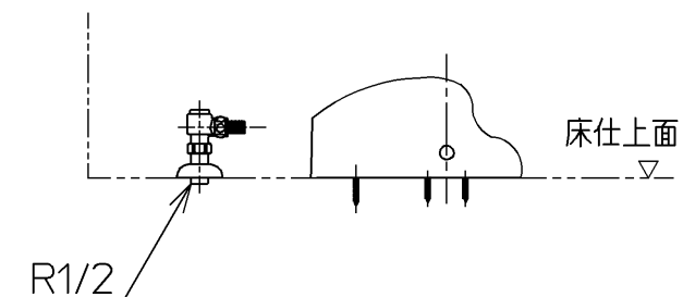
正面図
