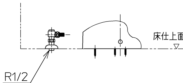
正面図
