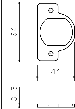
丁番用スペーサー(2ヶ)
