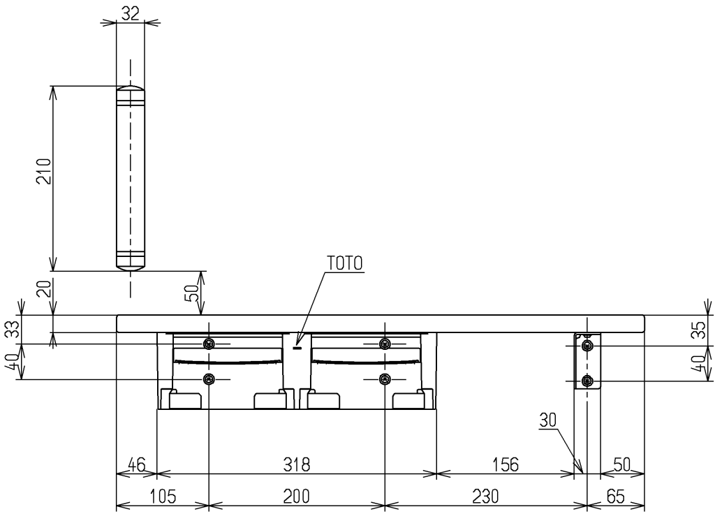
左壁設置の場合
