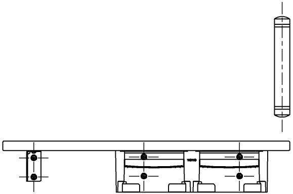
右壁設置の場合(1:8)
