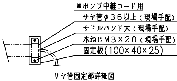
サヤ管固定部詳細図
