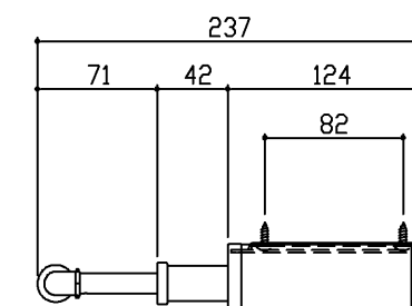
バーを最長に引き出した場合
