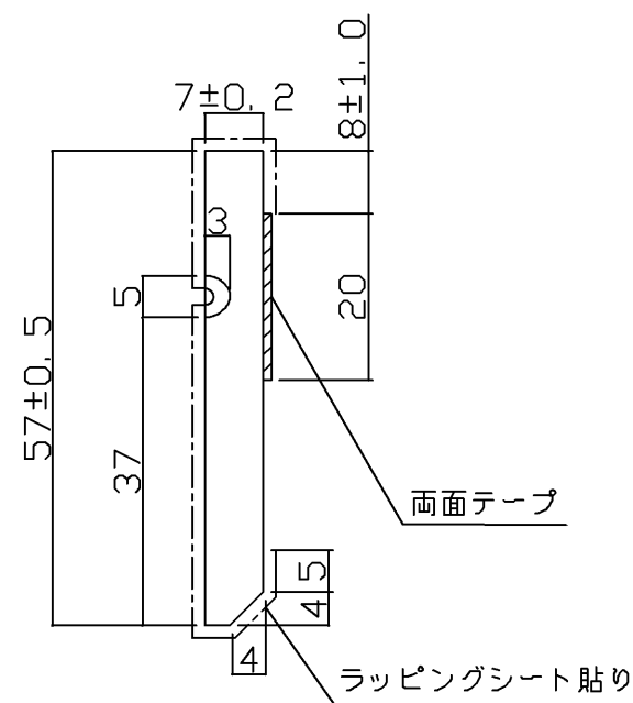
A-A断面図（1：1）
