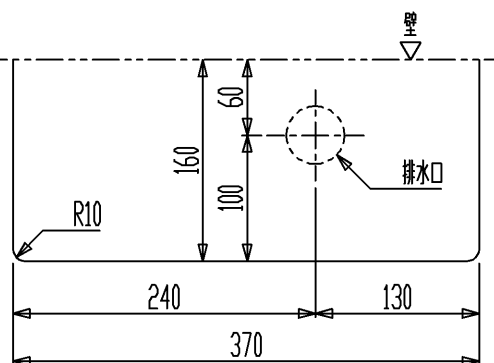
カウンター切込寸法 ※壁に寄せて設置する場合
