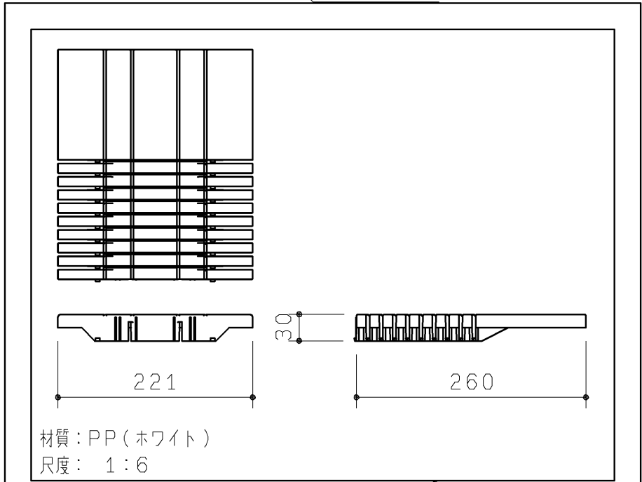
棚板（2ヶ）
