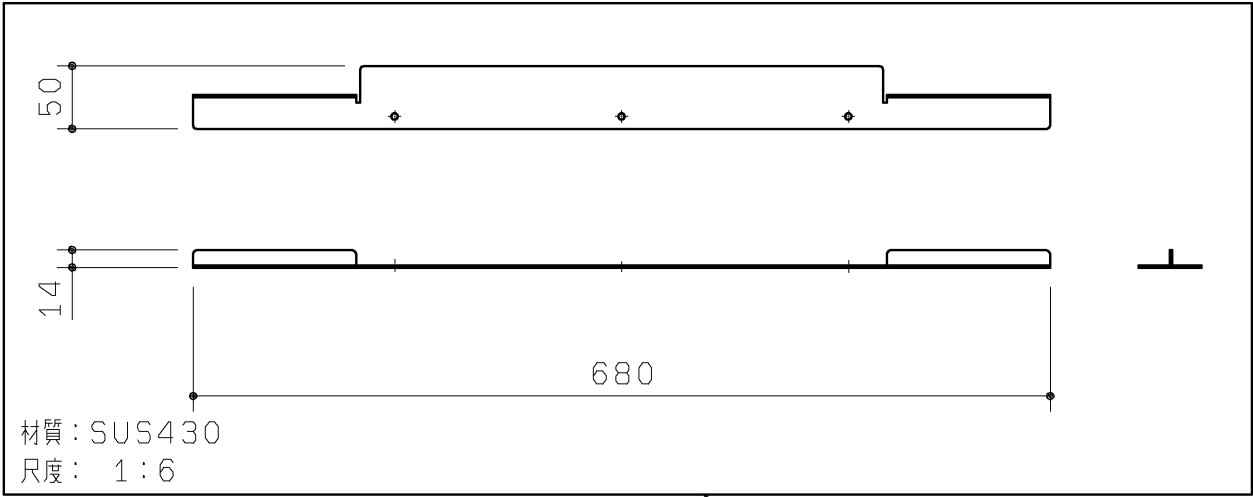
底板支持材
