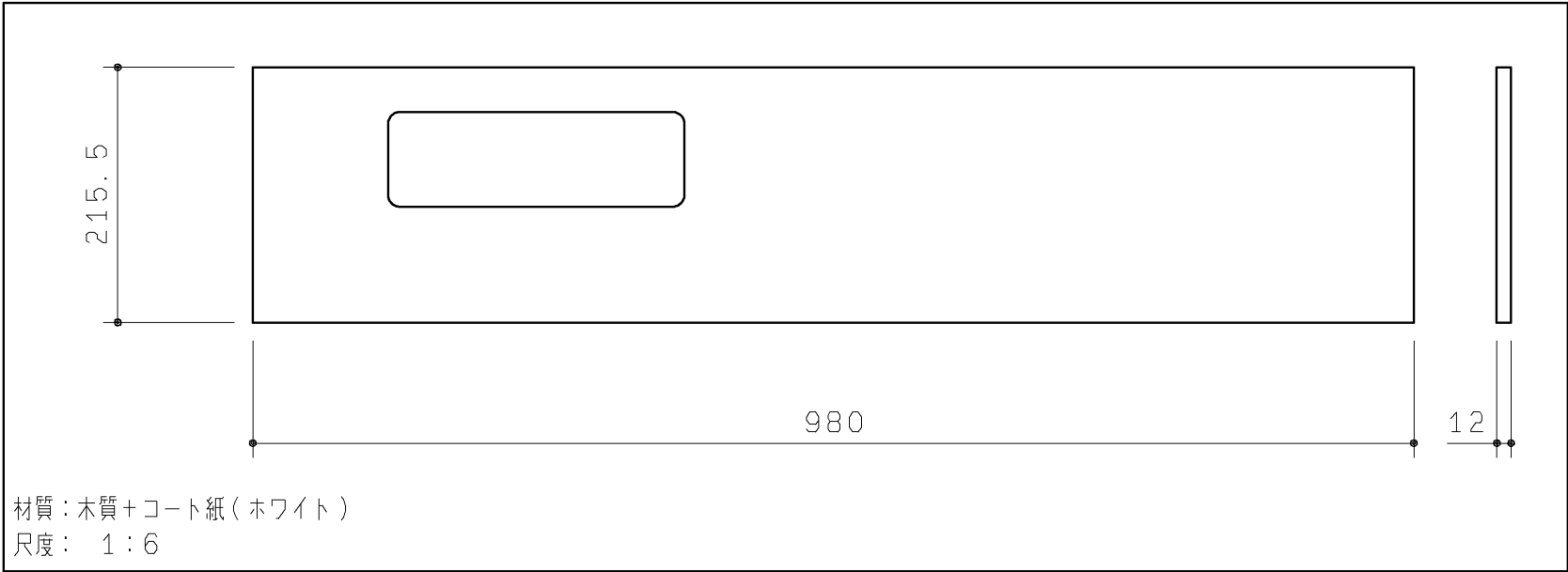
収納底板
